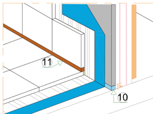
Detalhe juntas piso cerâmico
