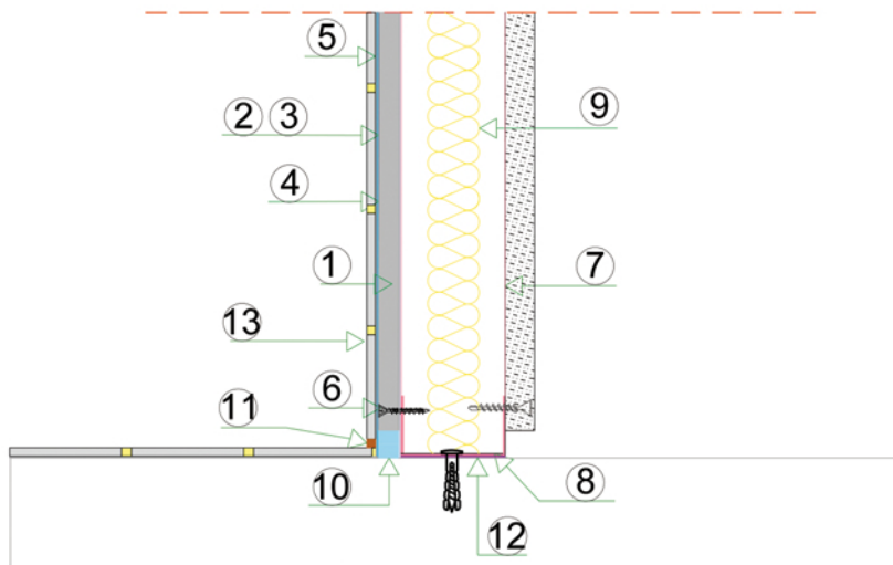
Detalhe juntas piso cerâmico
